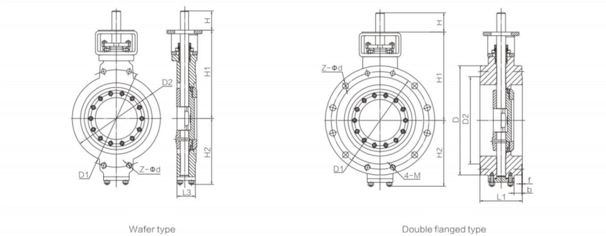
主要连接尺寸 (PN10.0MPa) Main connecting dimensions
