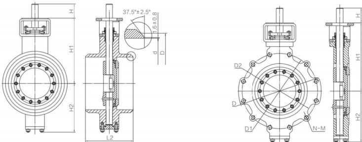
Butt weld type Lug type
