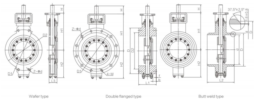
主要连接尺寸 (PN6.3MPa) Main connecting dimensions
