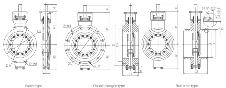
主要连接尺寸 (PN4.0MPa) Main connecting dimensions
