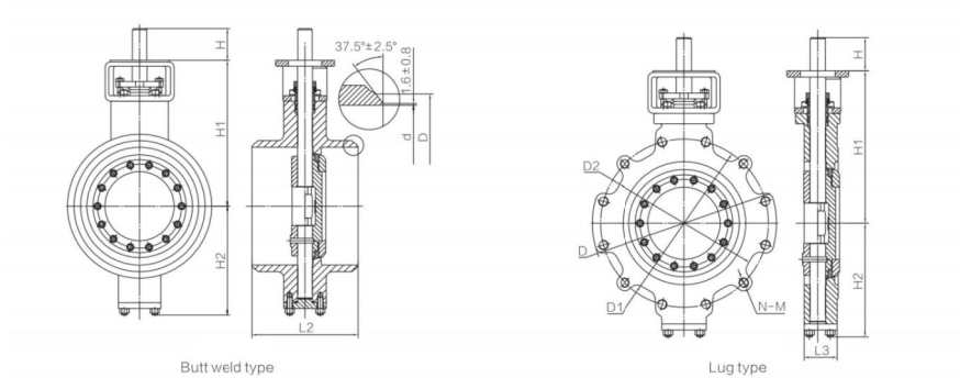
主要连接尺寸（600LB） Main connecting dimensions
