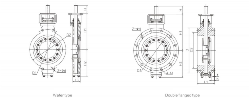
主要连接尺寸（300LB） Main connecting dimensions
