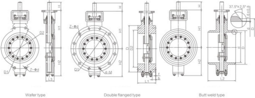
主要连接尺寸 (PN1.0 MPa) Main connecting dimensions
